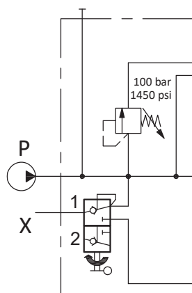
Left inlet
